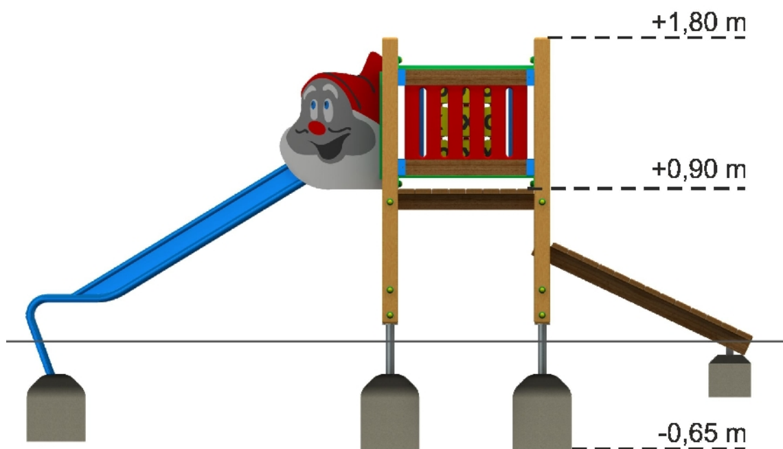
Rys. 6 Zjeżdżalnia mała (widok z boku - z wysokościami).
